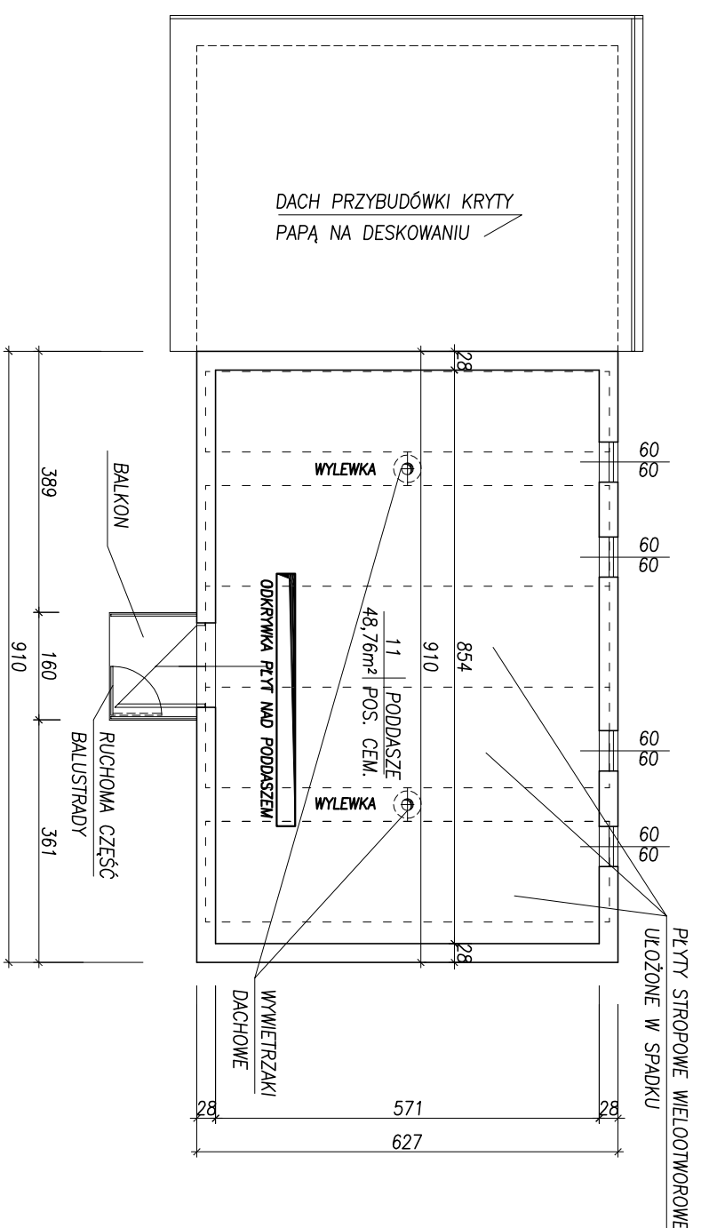
RZUT PODDASZA 1 : 100
