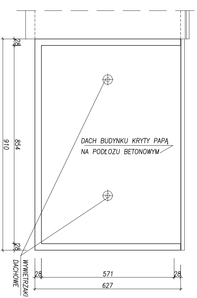
RZUT DACHU 1 : 100
