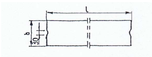
Rys. 1. Wymiarowanie krawężników
